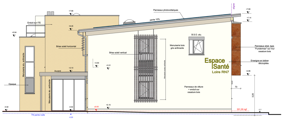
FACADE SUD-EST
