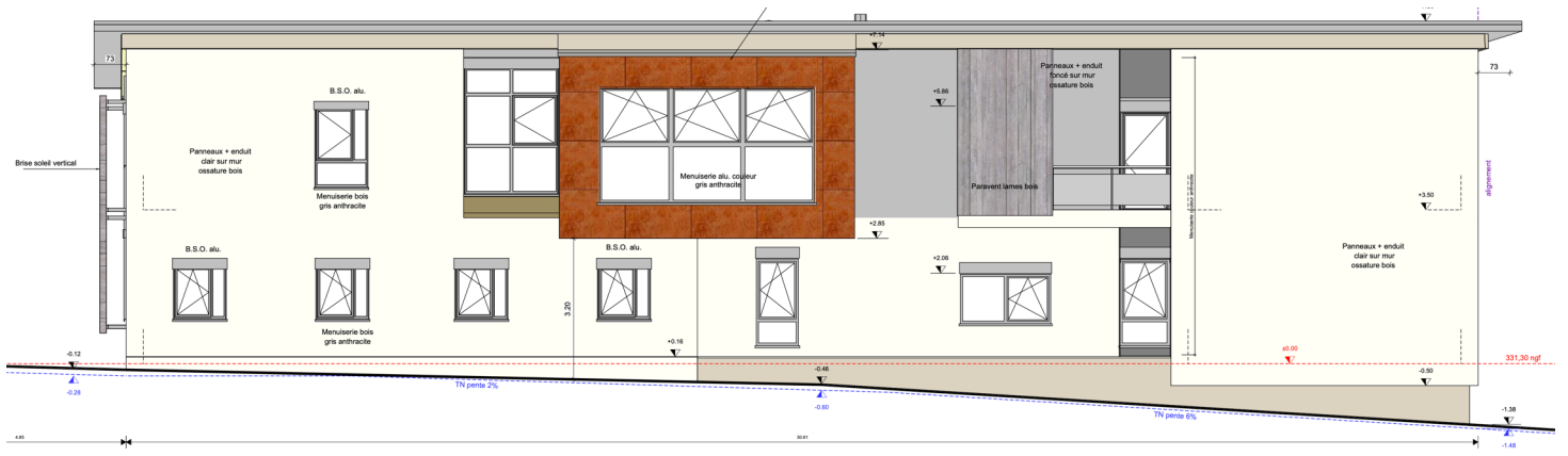
FACADE NORD-EST
