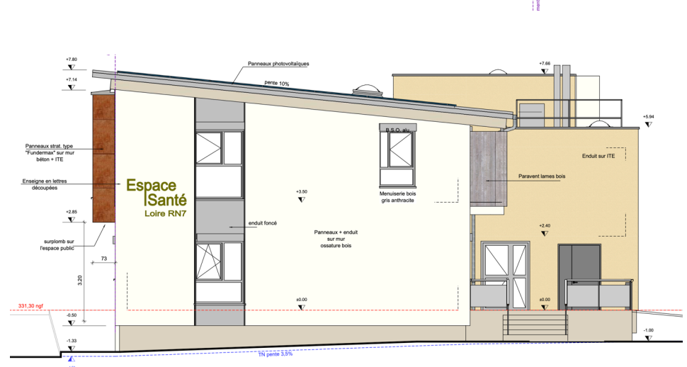
FACADE NORD-OUEST
